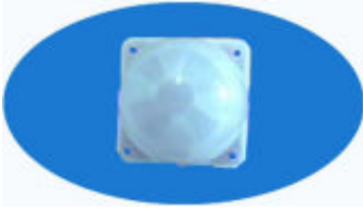
Type : 8002-1 focus : 10.5 angle : 100 ° distance : 5m dimension : 23
